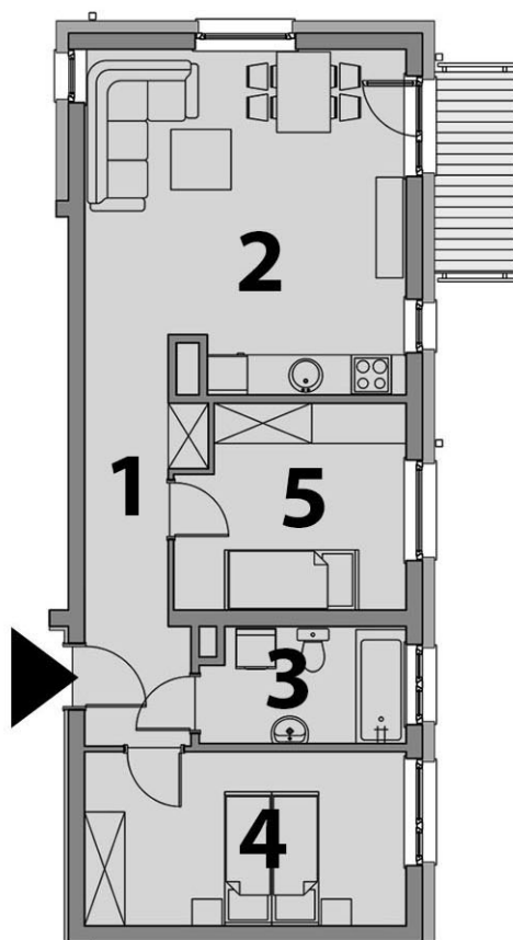
RZUTY KONDYGNACJI: PIĘTRO I
